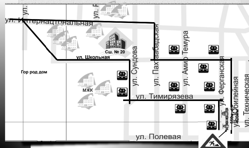
Схема водопроводных линий (замена трубы по ул Ферганской г Ош, протяж. 550м, сумма 8 200$)
